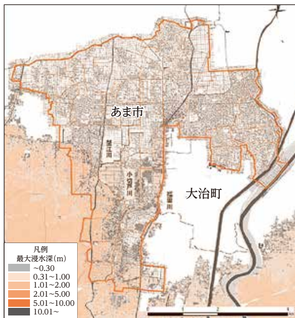
図2 津波最大浸水深分布図
